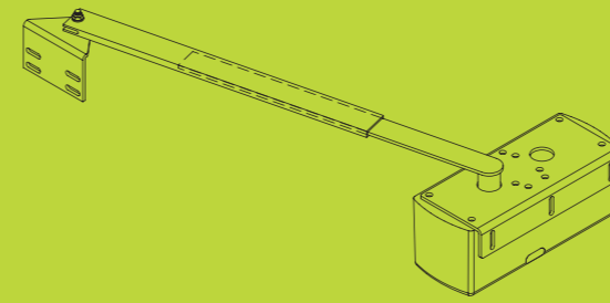
Particolare dell'automazione per portoni a libro a 2 ante. Detail of automation for double folding doors with 2 leaves.
