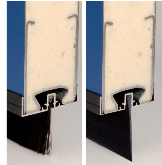
Spazzolini in nylon antiusura posti nei lati superiore ed inferiore dell'anta, montati su profilo in alluminio verniciato nero. Nylon brushes, wear-proof, placed on the top and the bottom edges of each door leaf, mounted on black aluminium profile.
