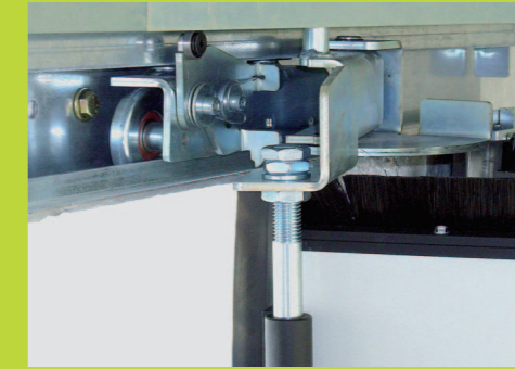
Dettaglio del carrello con deragliatore superiore per rotazione pacco 180° (Pat. Pend.). Detail of the carriage with top deviator for 180 degrees rotation (Pat. Pend.).
