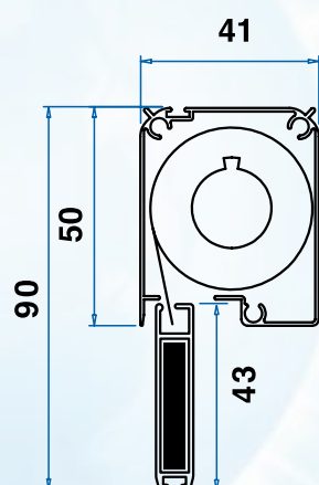
Cassonetto con tubo, rete e barra maniglia
