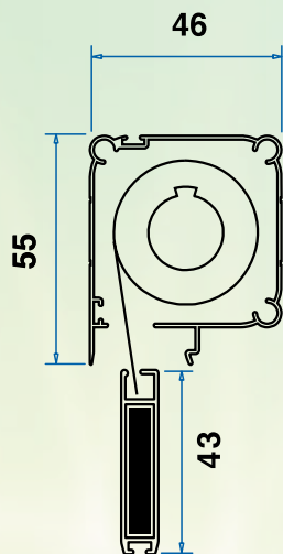
Cassonetto con tubo, rete, barra maniglia e contrappeso interno
