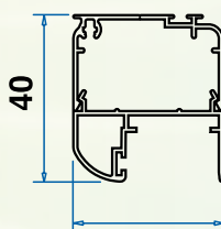
Profilo "U" e profilo copri "U"
