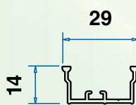
Barra di riscontro (per anta singola)
