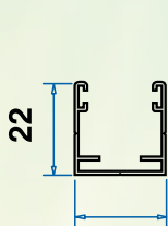
Guida a terra 22x22
