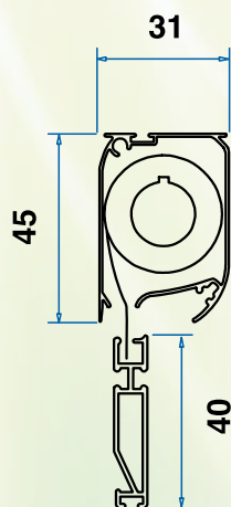
Cassonetto con tubo, rete e barra maniglia
