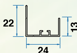
Profilo opzionale inferiore, consigliato per il modello a catenella e per tutte le installazioni frontali.
