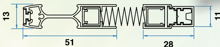
Barra maniglia + guida laterale (anta singola)
