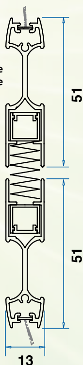
Barra maniglia e pacchetto rete
