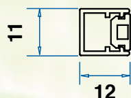
Barra di riscontro
