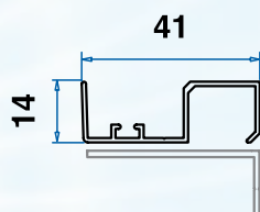
Barra di riscontro* (vedi nota a lato)
