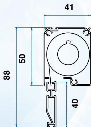
Cassonetto con tubo, rete e barra maniglia
