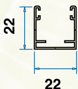
Guida a terra 22x22
